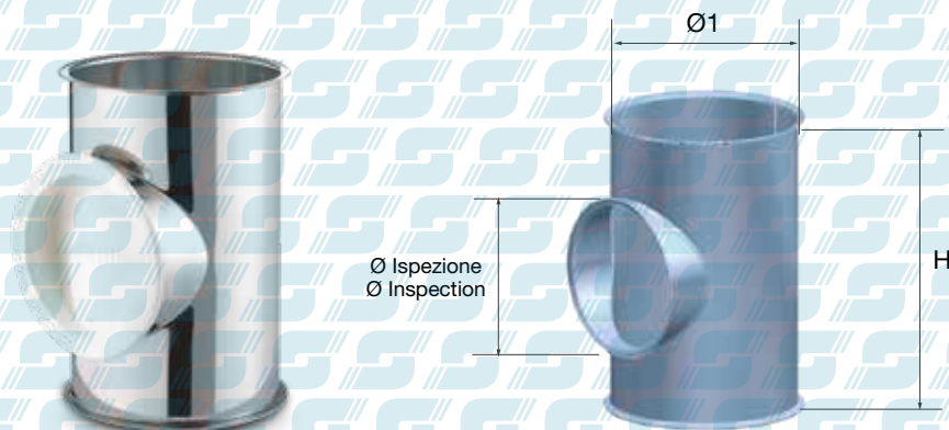
Tubi di Ispezione 90° - Inspection spouts 90°
