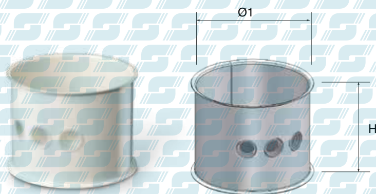
Prese d'aria con fori - False air inlet with holes
